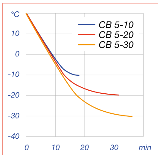
Curva di raffreddamento
